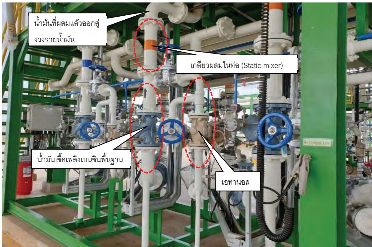
ตัวอย่าง ระบบท่อที่ใช้ในการในการผสมจ่ายน้ำมันแก๊สโซฮอล์ 91 ที่คลังน้ำมันศรีสะเกษ
